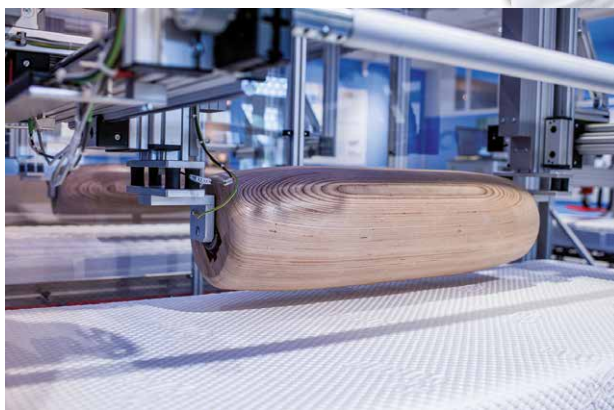
Testování mechanické odolnosti. Simulace životnosti matrace maximálním zatížením v nejexponovanější části matrace válcováním.
