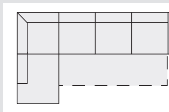
SPŘUP/L + SR + S3R/P š/307xh/211xv/93 lůžko 140 x 270
